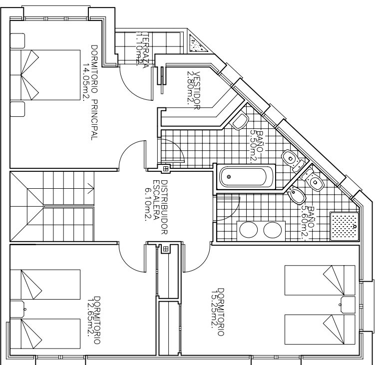
PLANTA PRIMERA
